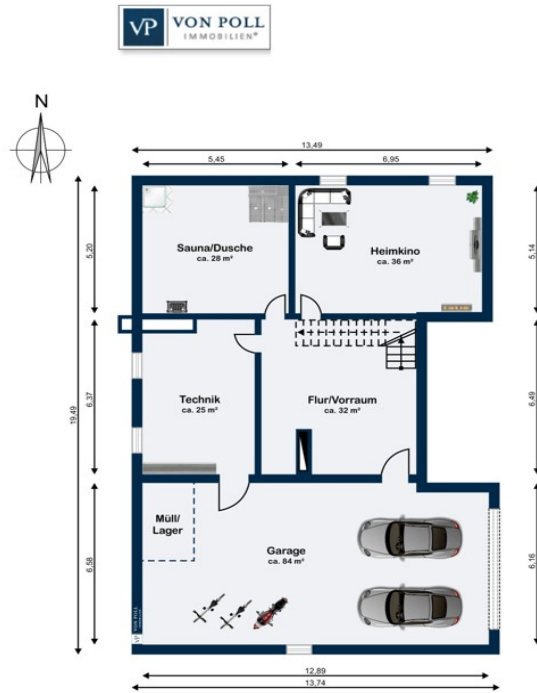
Kellergeschoss
