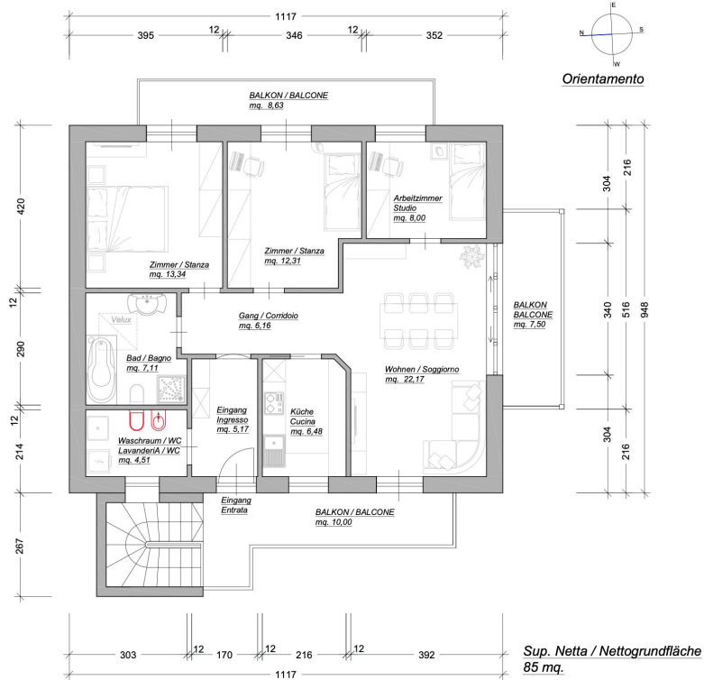
GRUNDRISS / PLANIMETRIA Variante 1 - mit WC im Waschraum / con WC in lavanderia
