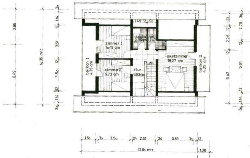
dachgeschoss
