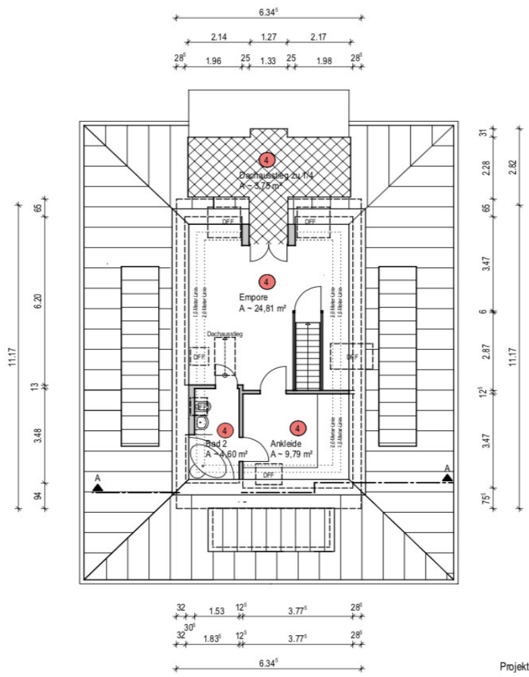
Grundriss 2. Dachgeschoss
