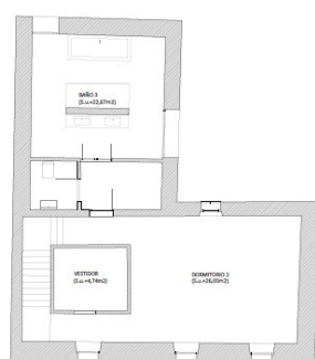
PIANTA PRIMITA - Scala 1/75
