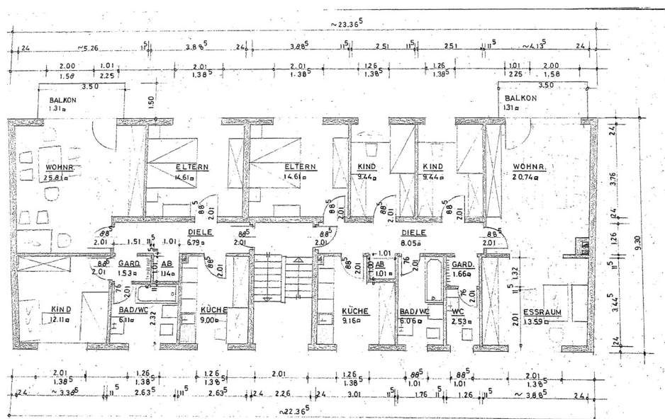
1.+2. OBERGESCHOSS M.1:100
