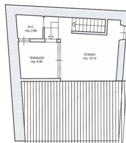
TERZO PIANO
