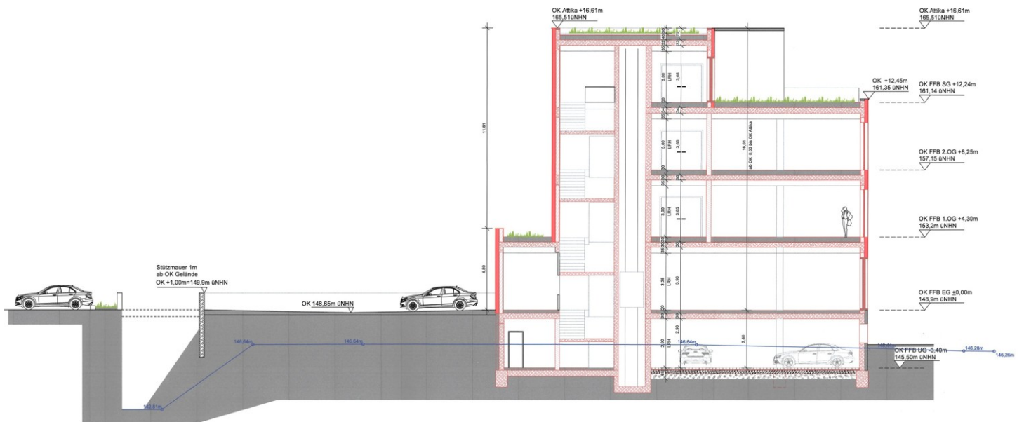
Schnitt C-C
