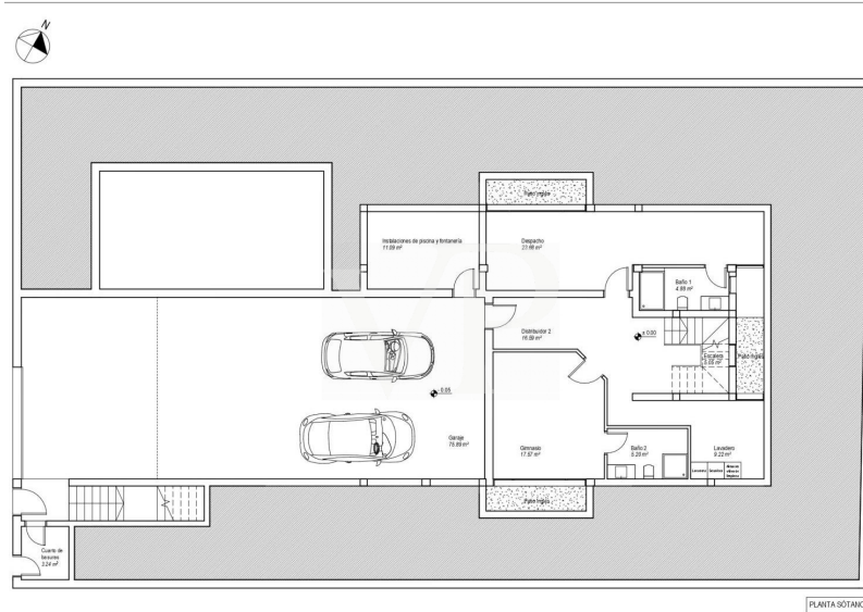
PLANTA SÓTANO
