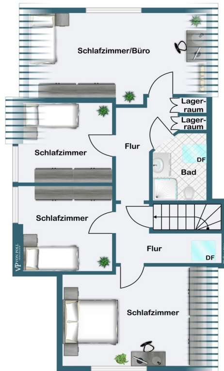
Dachgeschoss
