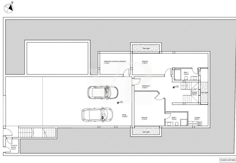
PLANTA SOTANO
