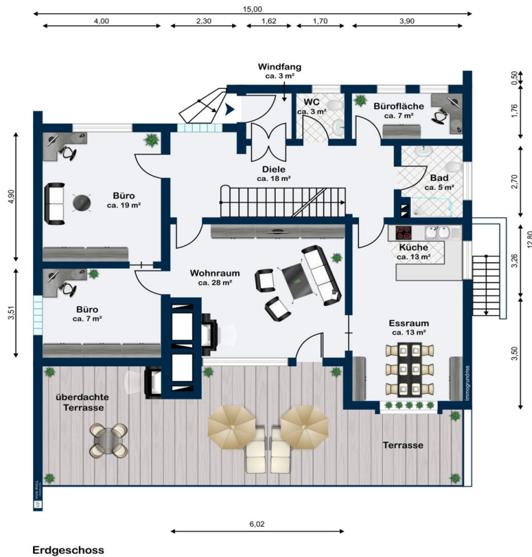
Erdgeschoss
