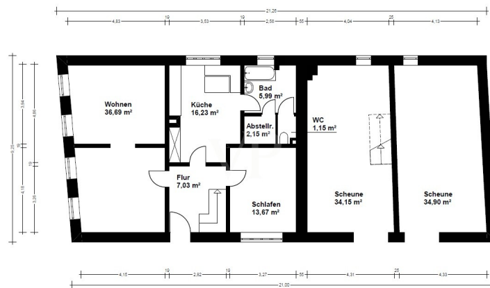
Grundriss EG
