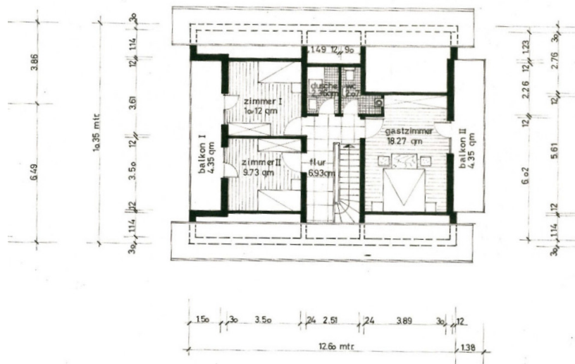
dachaeschoß
