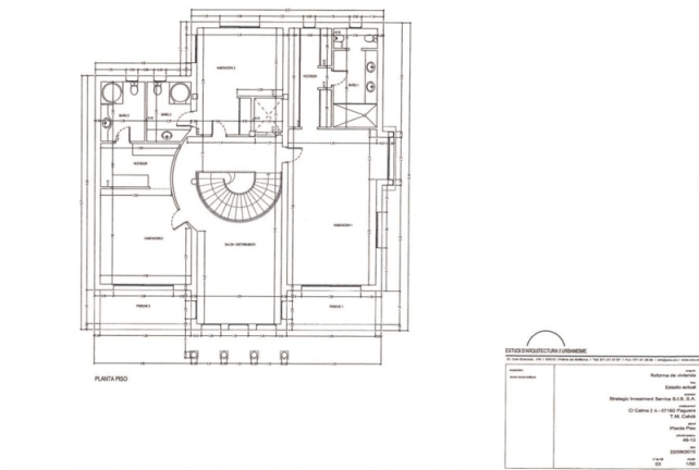
Grundriss Obergeschoss
