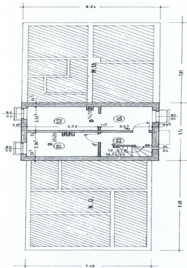
KELLERGESCHOSS GRUNDRISS
