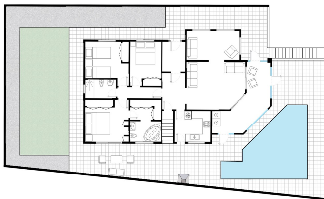
PLANTA BAJA
