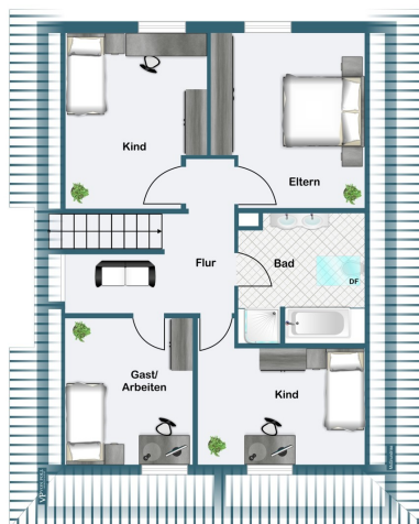
Obergeschoss
