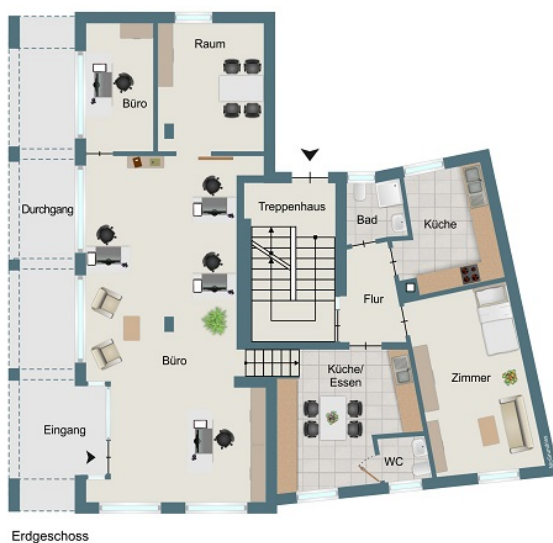
Erdgeschoss
