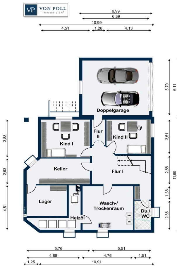
Kellergeschoss
